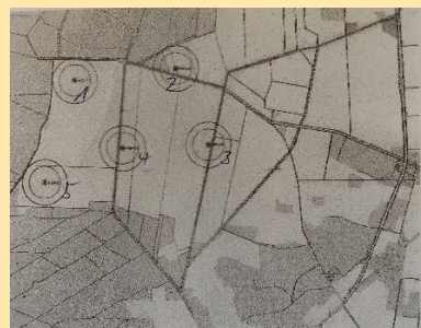
wpd geplante 5 Windräder
